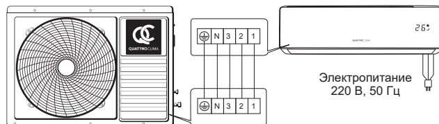
Электрическая схема QN-SR07...18WA / QV-SR07...18WA
