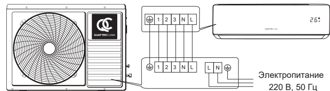
Электрическая схема QN-SR24WA / QV-SR24WA
