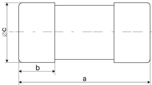
Рис. 1 Габаритные размеры плавких вставок ПВЦ
