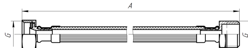
Рисунок 3 – Габаритные и присоединительные размеры подводки вн-нар
