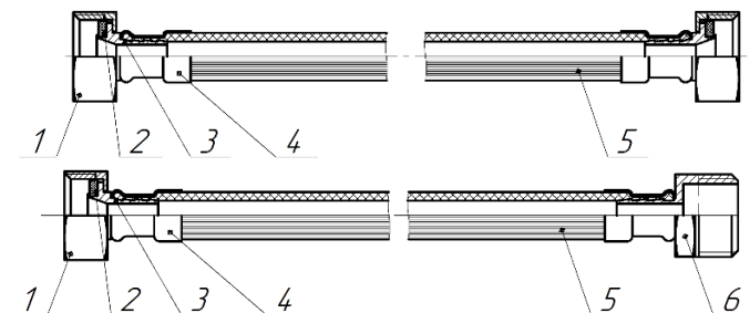
Рисунок 1 – Общий вид и конструкция изделия
