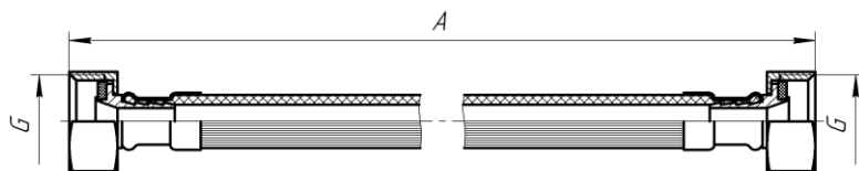
Рисунок 2 – Габаритные и присоединительные размеры подводки вн-вн
