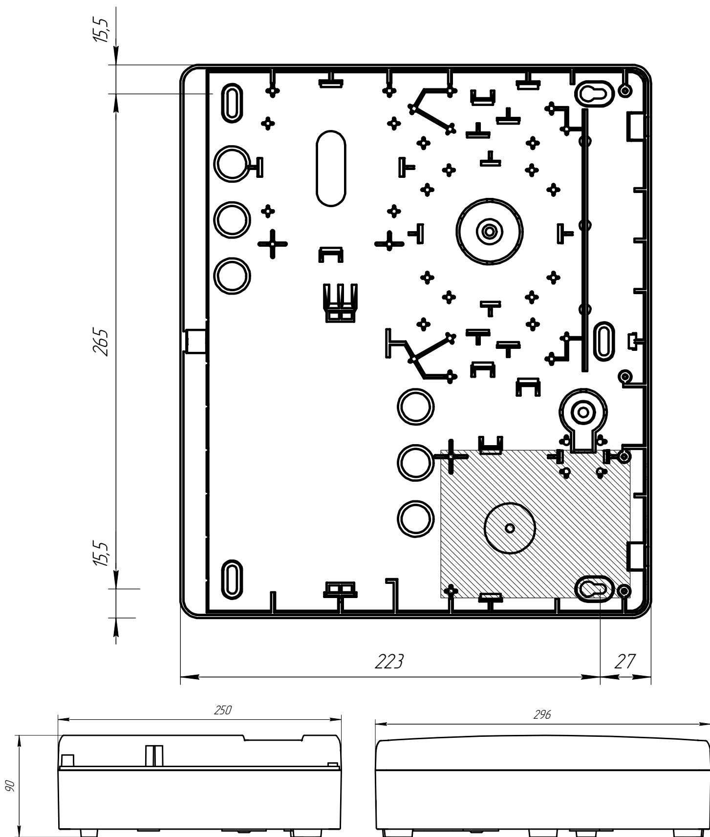
Рисунок 2. Корпус «Контакт» под АКБ 7 Ач
