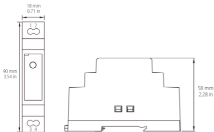
Рисунок 1. Внешний вид и обозначение клемм SMARTWATT PSE DR 1215 и 2415.
