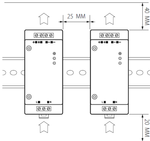
Рисунок 5. Размещение блока питания.
