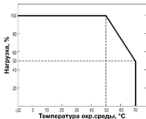
Рисунок 8. График зависимости нагрузочной способности блока питания от температуры окружающей среды.
