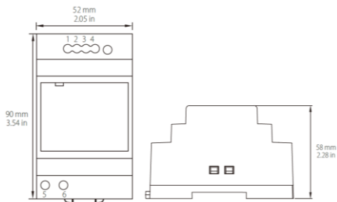
Рисунок 3. Внешний вид и обозначение клемм SMARTWATT PSE DR 1260, 2445 и 2460.
