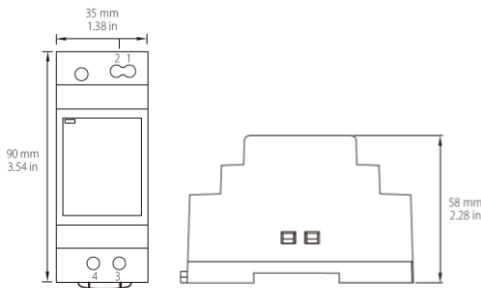
Рисунок 2. Внешний вид и обозначение клемм SMARTWATT PSE DR 1230 и 2430.
