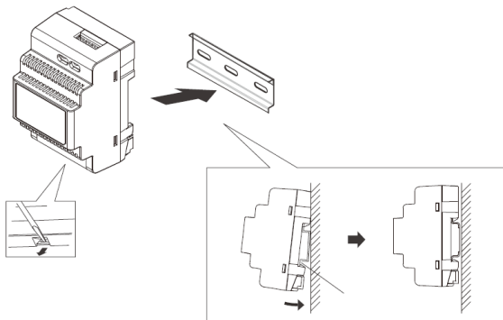
Рисунок 7. Установка блока питания на DIN-рейку.
