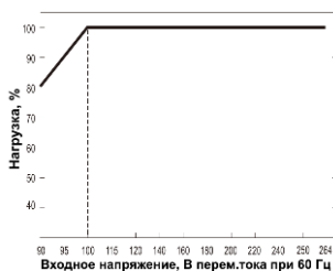
Рисунок 9. График зависимости нагрузочной способности блока питания от входного напряжения.
