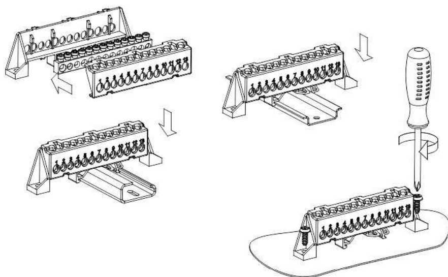
а) шина в комбинированном DIN-изоляторе «Стойка»
