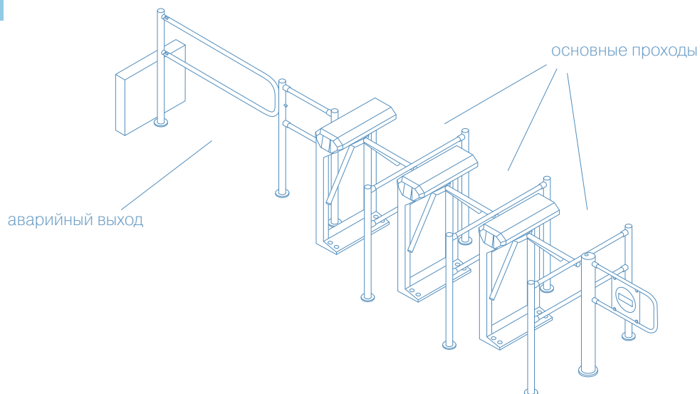
Электронные проходные со стандартными и поворотной секциями ограждений, калитка
