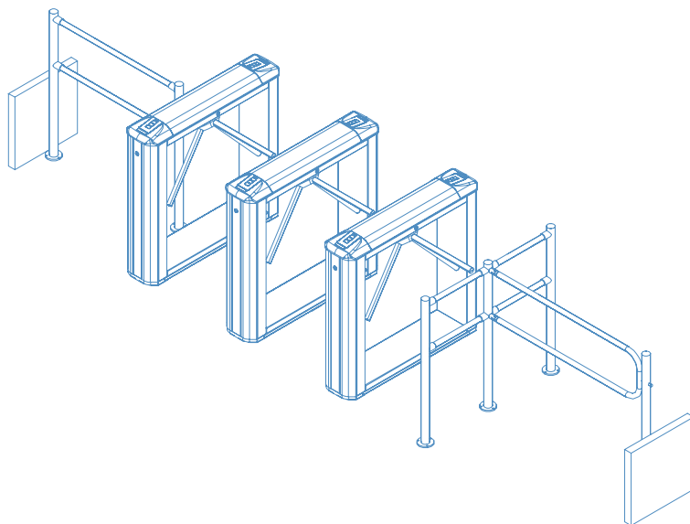
Электронные проходные со стандартными и поворотной секциями ограждений
