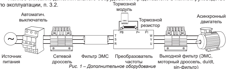
Рис. 1 – Дополнительное оборудование
