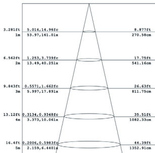
Диаграмма распределения светового потока и диаграмма освещенности
