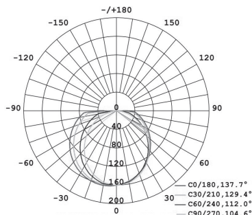
Диаграмма распределения светового потока и диаграмма освещенности
