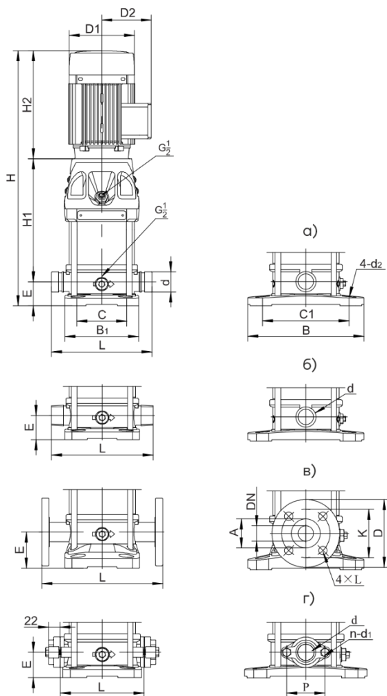
Рисунок 8 - Габаритно-присоединительные размеры а) viciatic (группа); б) трубная резьба; в) DIN-фланец; г) овальный фланец
