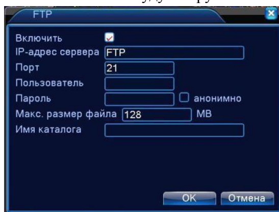
Рисунок 4.23 Настройки FTP
