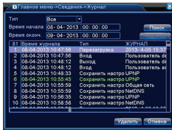
Рисунок 4.54 Информация журнала
