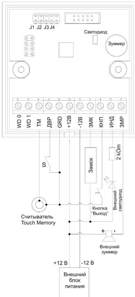
Рисунок 2 – Подключение СКУД со считывателем Touch Memory
