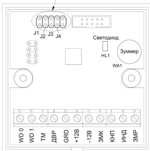
Рисунок 4 – Программирование с помощью перемычек (джамперов). выбрать режим и замкнуть перемычкой
