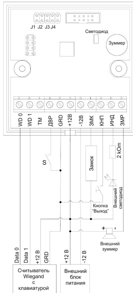
Рисунок 3 - Подключение СКУД со считывателем Wiegand
